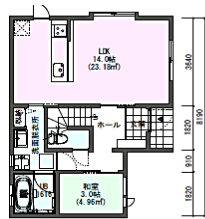
1階
